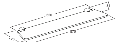
Valencia Glass Shelf - 75680A-CP
